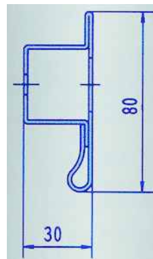
verzinkt stalen profiel
