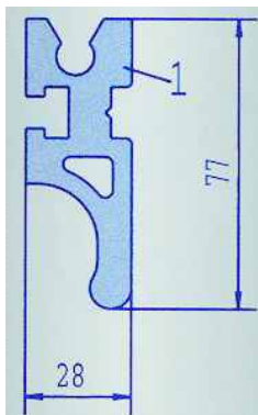
aluminiumprofiel
